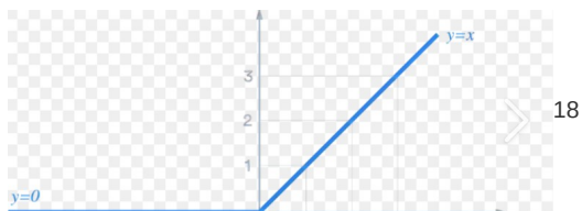
Abbildung 54: Relu-Schicht
