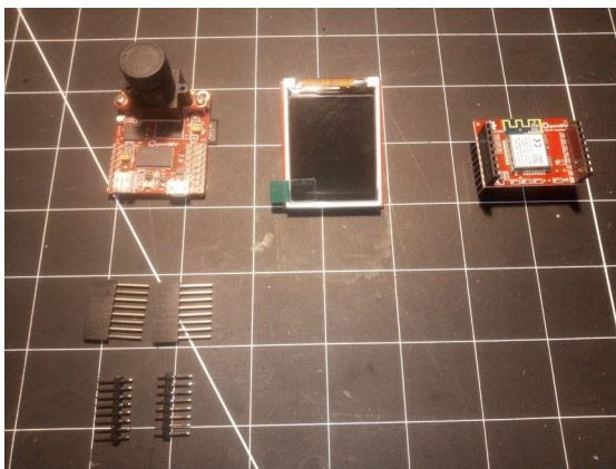
Abbildung 10: Einzelkomponenten Vorderseite
